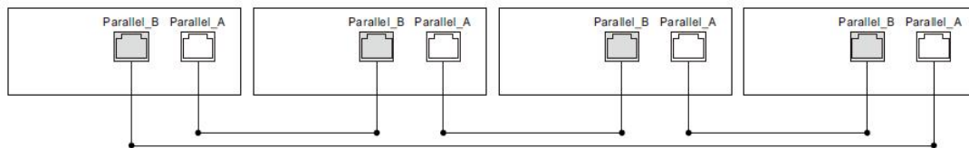
d) 系统五台逆控一体机并联：
