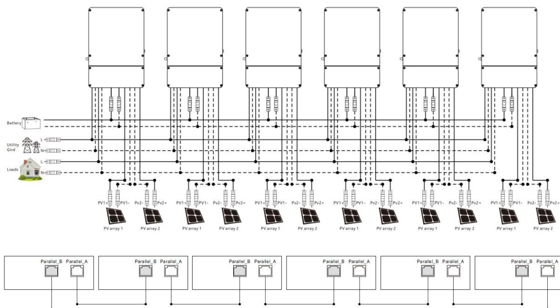
e) 系统六台逆控一体机并联：
